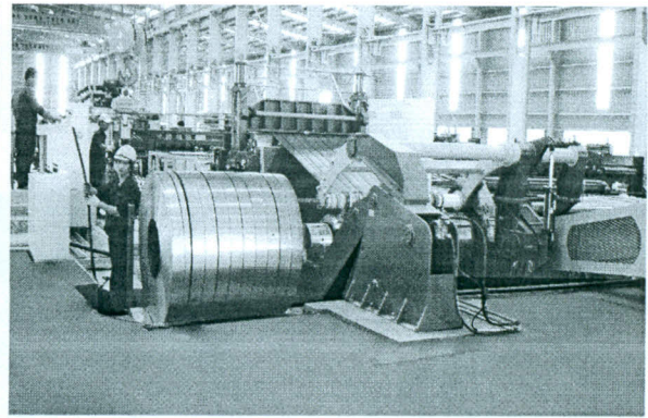
Hình 2: Dây chuyền xẻ băng
